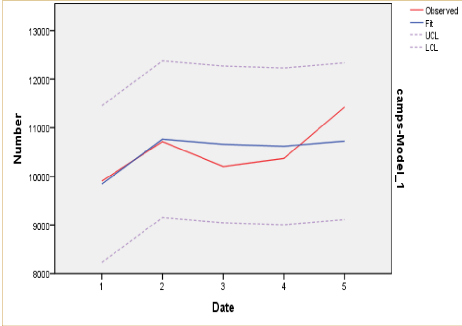
شكل (٨) يبين منحني المشاهدات الاصلية للسلسلة الزمنية ومنحنى القيم التنبؤية
